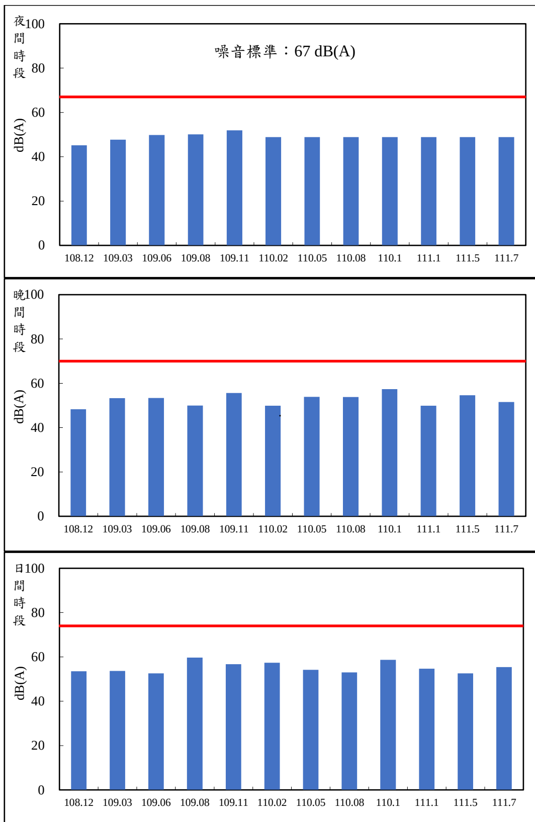
圖 3.1.14-3 歷次中港慈裕宮噪音監測結果變化情形
