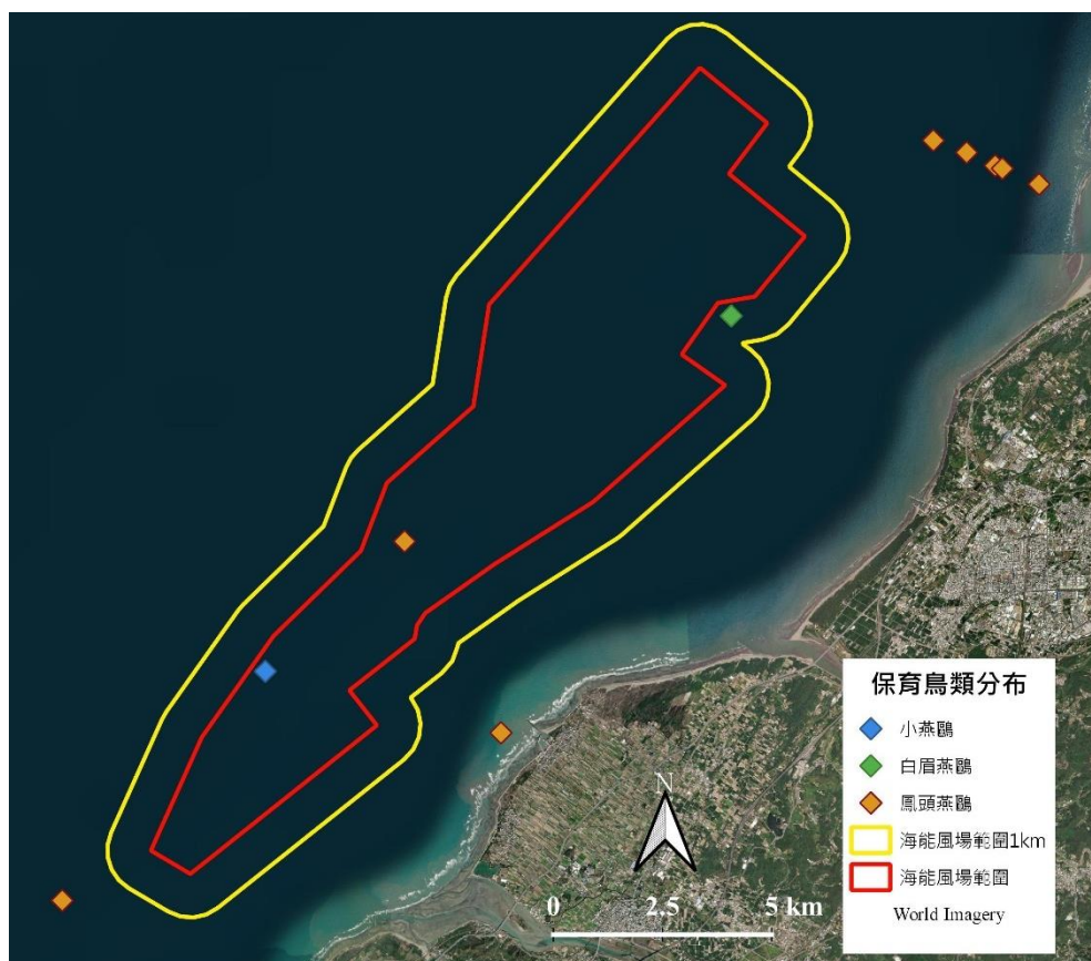
圖 2.1.1-1 海上保育類鳥類分布
