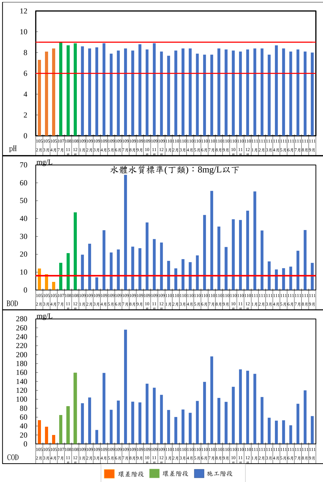
圖 3.1.15-1 歷次竹南人工暫定重要濕地水質監測結果變化情形
