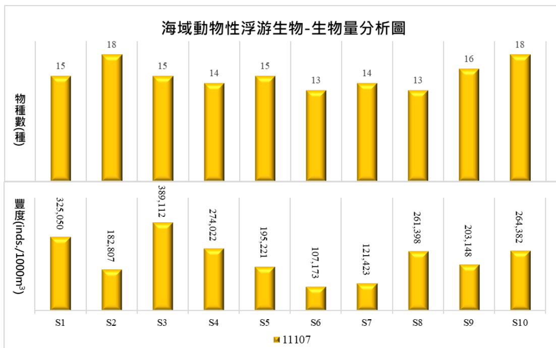
圖 2.1.9-3 動物性浮游生物生物量分析圖
