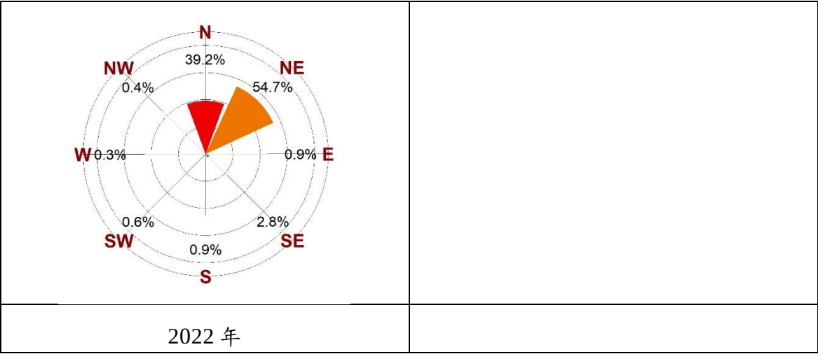
圖 3.1.1-1 歷年春季鳥類飛行方向風花圖
