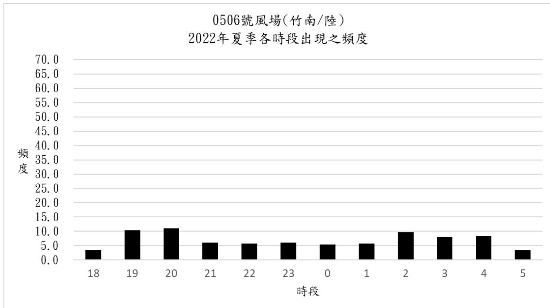
圖 2.1.2-4 夜間鳥類飛行活動模式(竹南測站)
