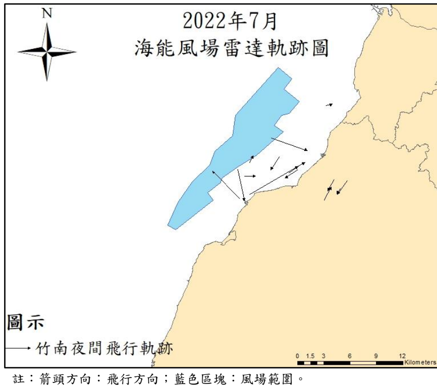
圖 2.1.2-7 2022 年 7 月 竹南測站夜間鳥類飛行軌跡
