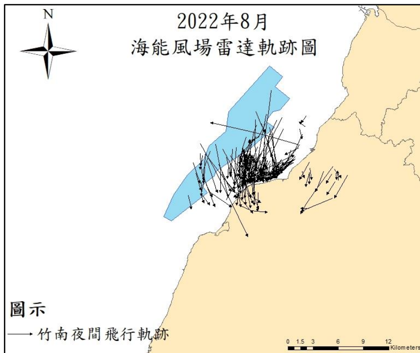
圖 2.1.2-8 2022 年 8 月 竹南測站夜間鳥類飛行軌跡
