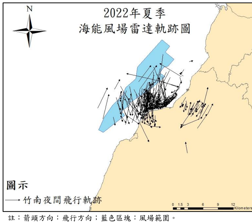
圖 2.1.2-5 2022 夏季竹南測站夜間鳥類飛行軌跡
