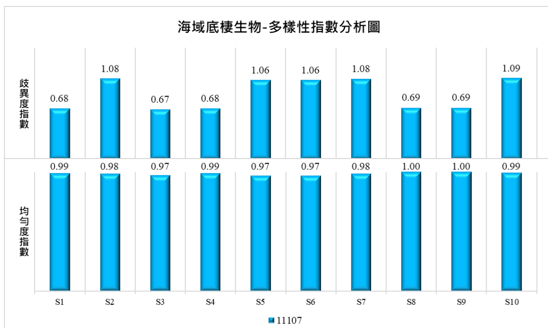
圖 2.1.9-6 海域底棲生物多樣性指數分析圖
