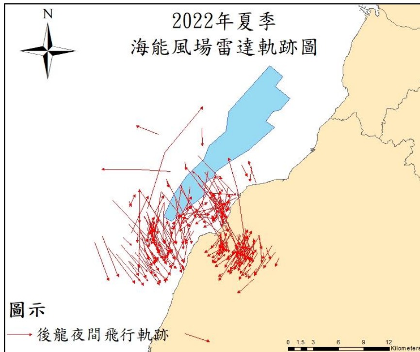
圖 2.1.2-11 2022 夏季後龍測站夜間鳥類飛行軌跡
