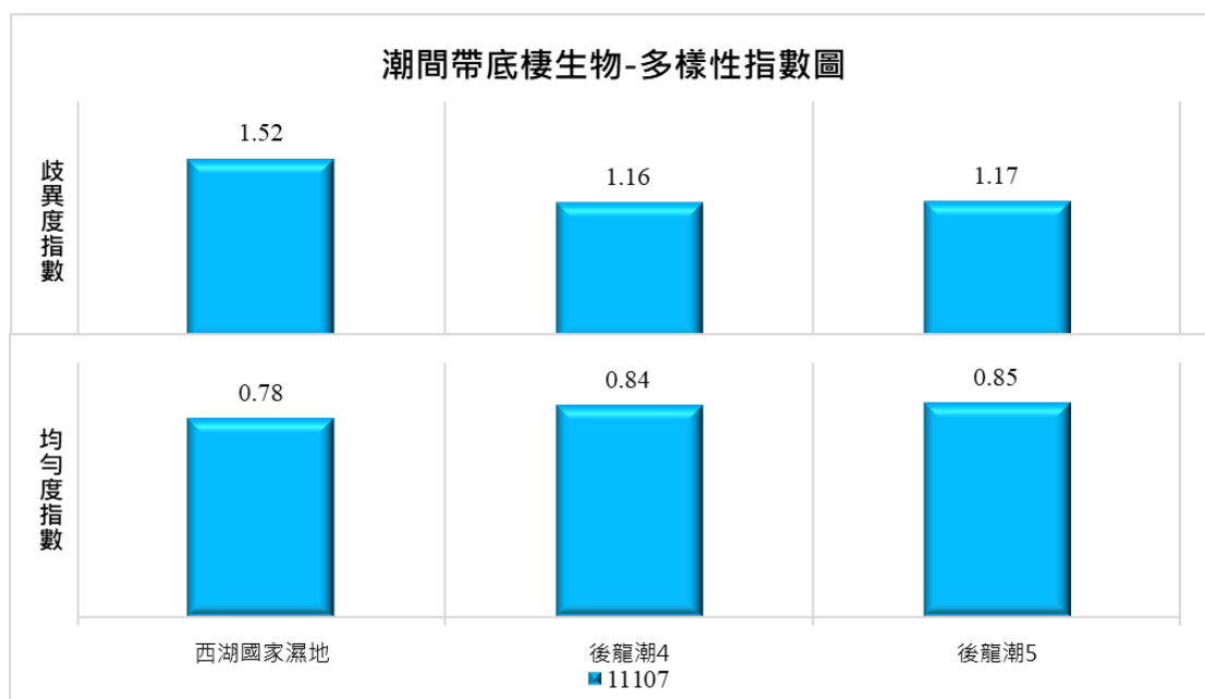
圖 2.1.9-8 底棲生物多樣性指數分析圖
