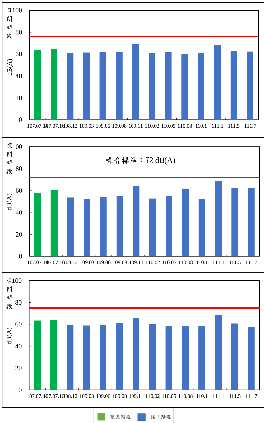
圖 3.1.14-2 歷次陸纜沿線民宅噪音監測結果變化情形
