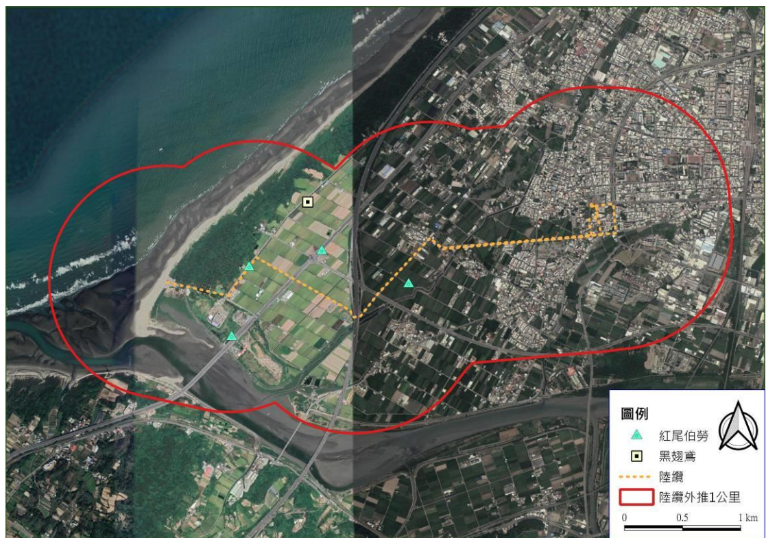
圖 3.1.10-9 施工階段-2021 年秋季保育鳥種分布圖
