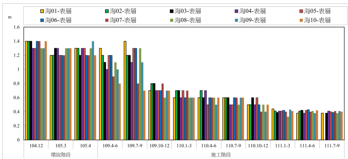
圖 3.1.7-3 歷次透明度變化圖
