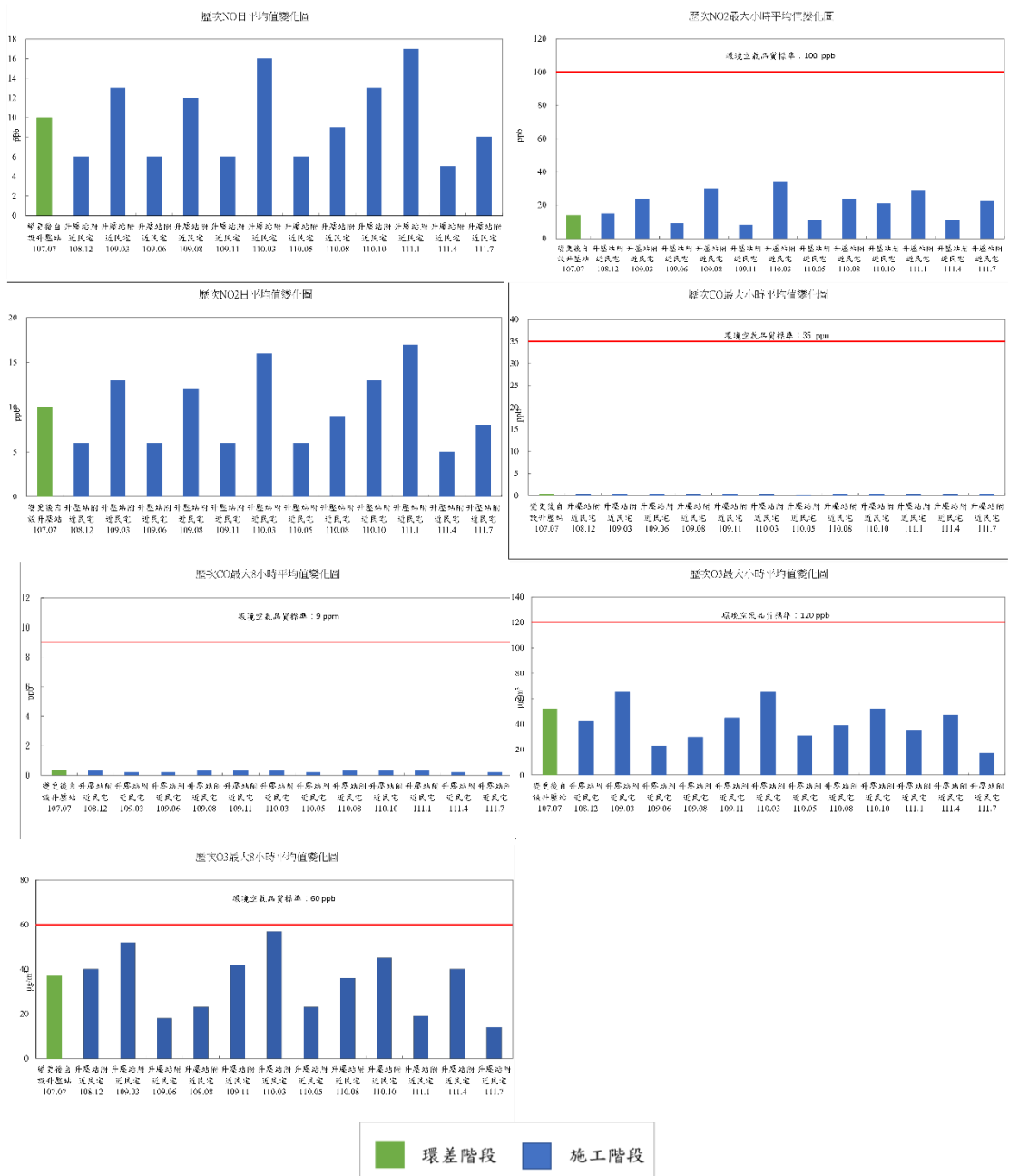
圖 3.1.13 環差及監測階段-歷次空氣品質變化圖(續)
