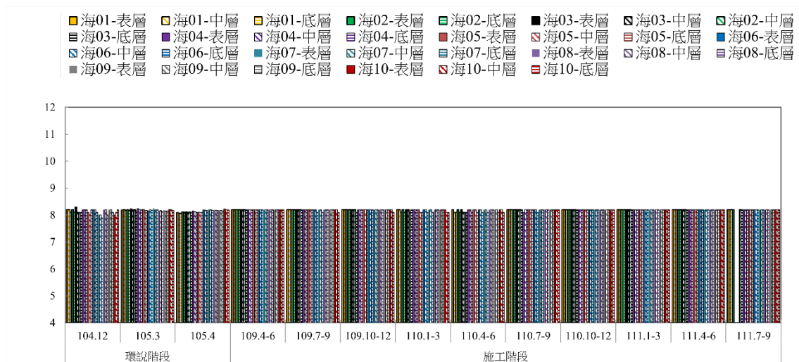
圖 3.1.7-1 歷次 pH 值變化圖
