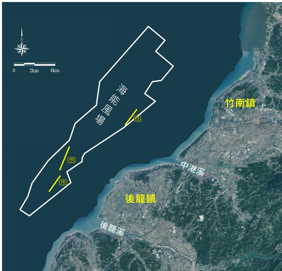
圖 1.3.3-4 魚類調查測線位置圖
