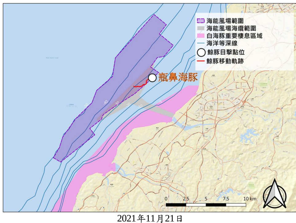
圖 3.1.3-5 施工階段-2021 年度鯨豚調查目擊點位與軌跡記錄
