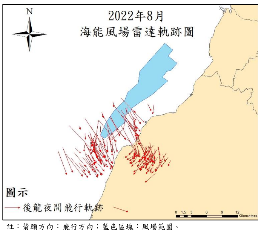
圖 2.1.2-14 2022 年 8 月後龍測站夜間鳥類飛行軌跡
