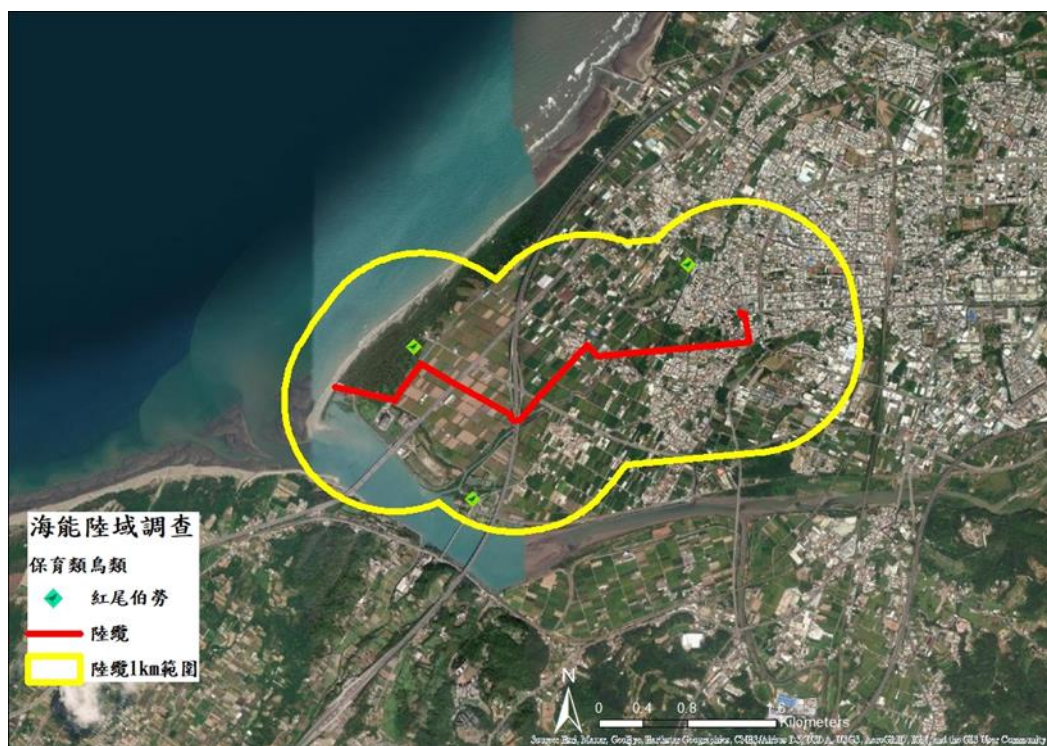
圖 3.1.10-6 施工階段-2020 年秋季保育鳥種分布圖
