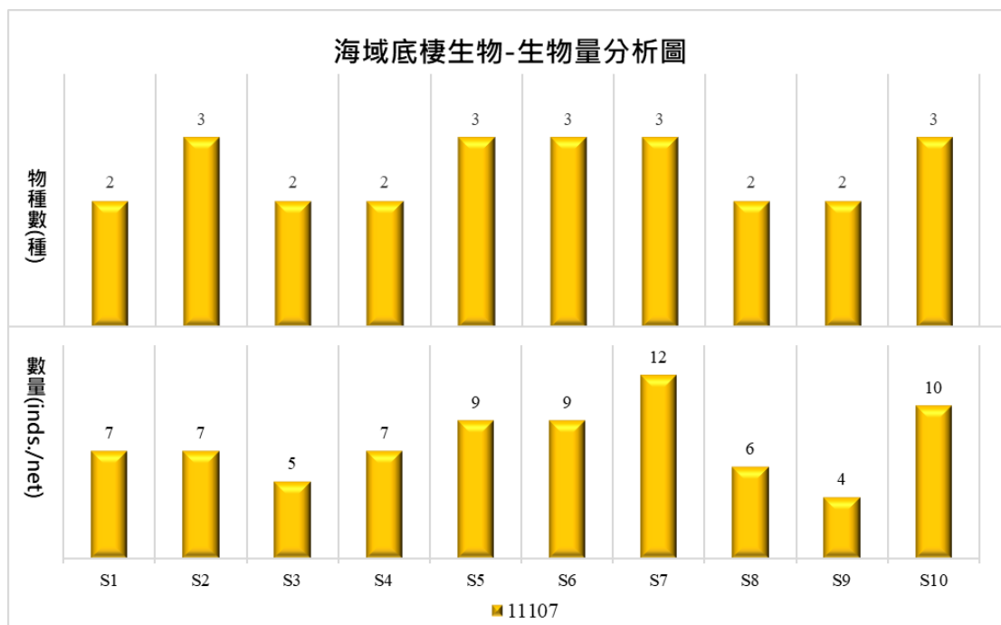
圖 2.1.9-5 海域底棲生物生物量分析圖
