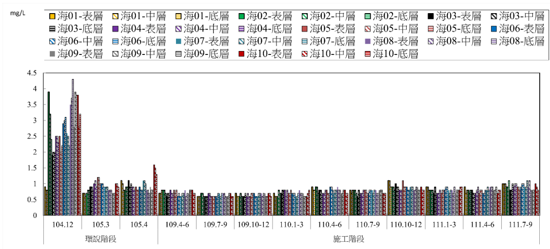
圖 3.1.7-5 歷次生化需氧量變化圖
