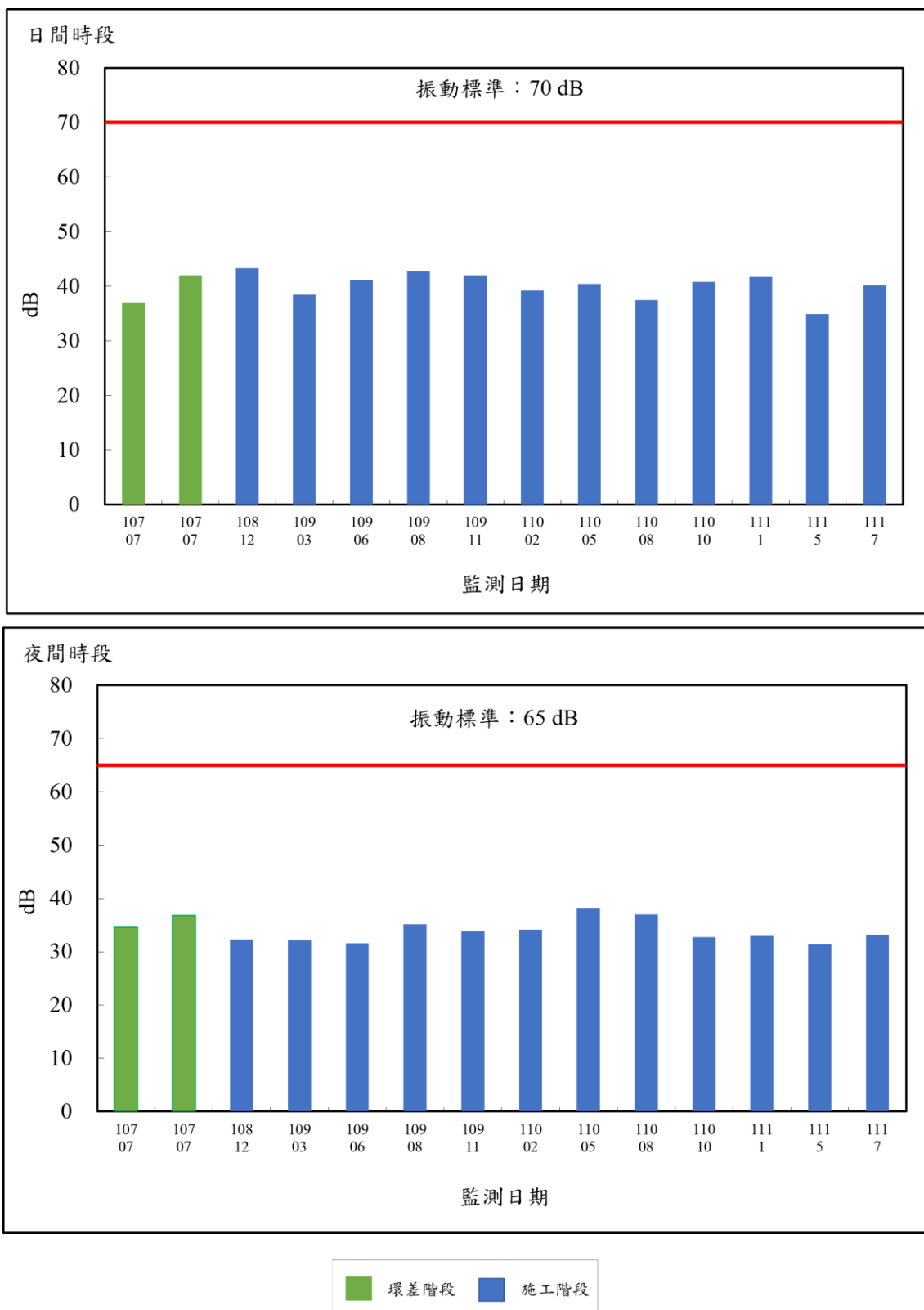
圖 3.1.14-5 陸纜沿線民宅振動監測結果變化情形
