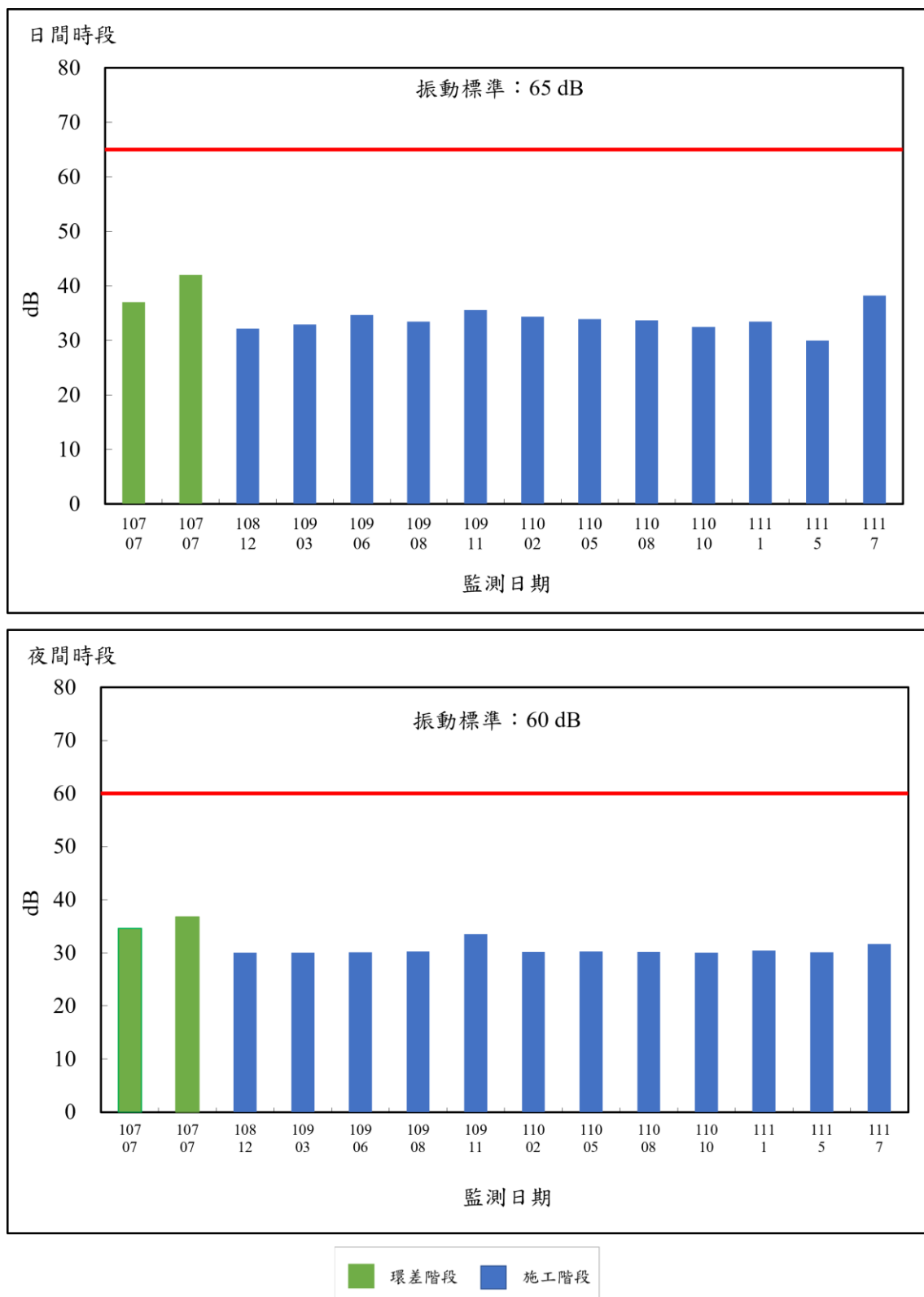
圖 3.1.14-4 升壓站附近民宅振動監測結果變化情形
