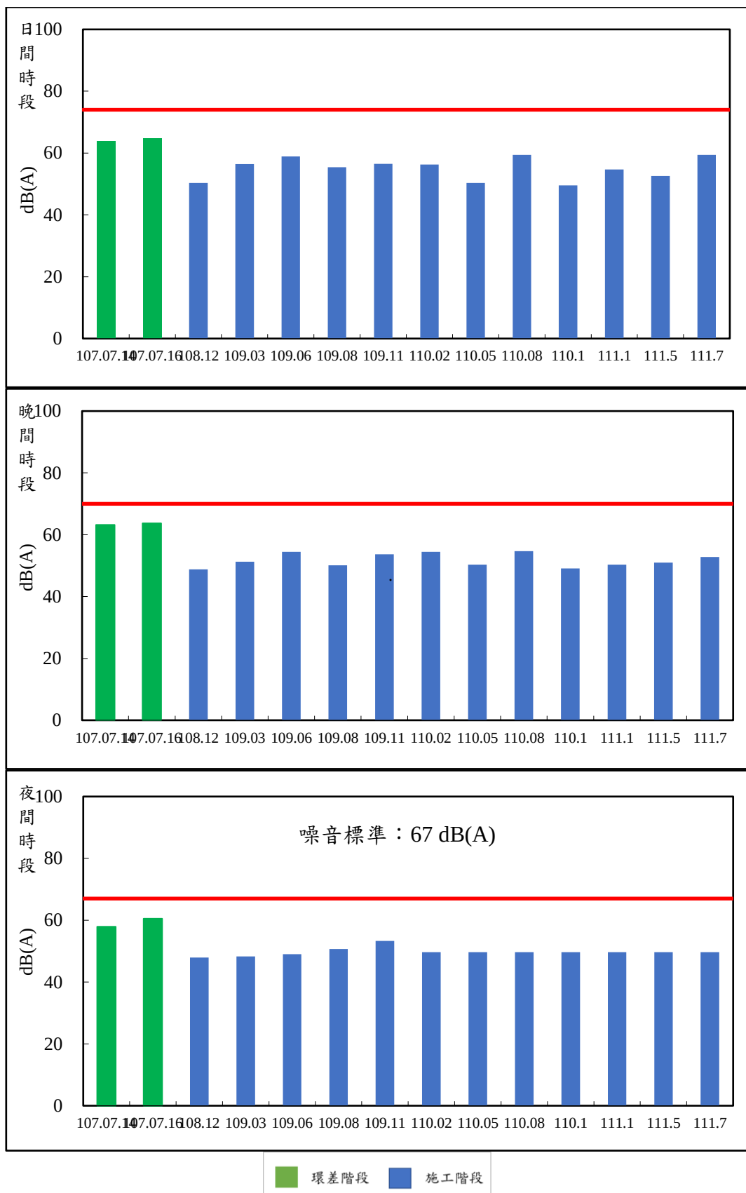
圖 3.1.14-1 歷次升壓站附近民宅噪音監測結果變化情形
