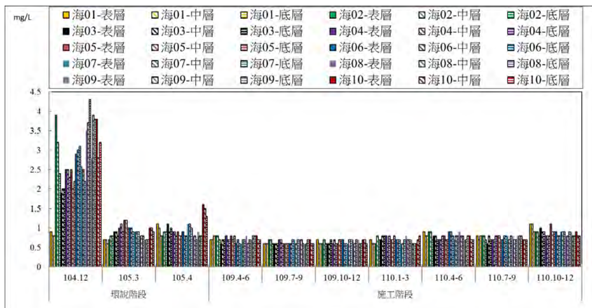
圖 3.1.7-5 歷次生化需氧量變化圖
