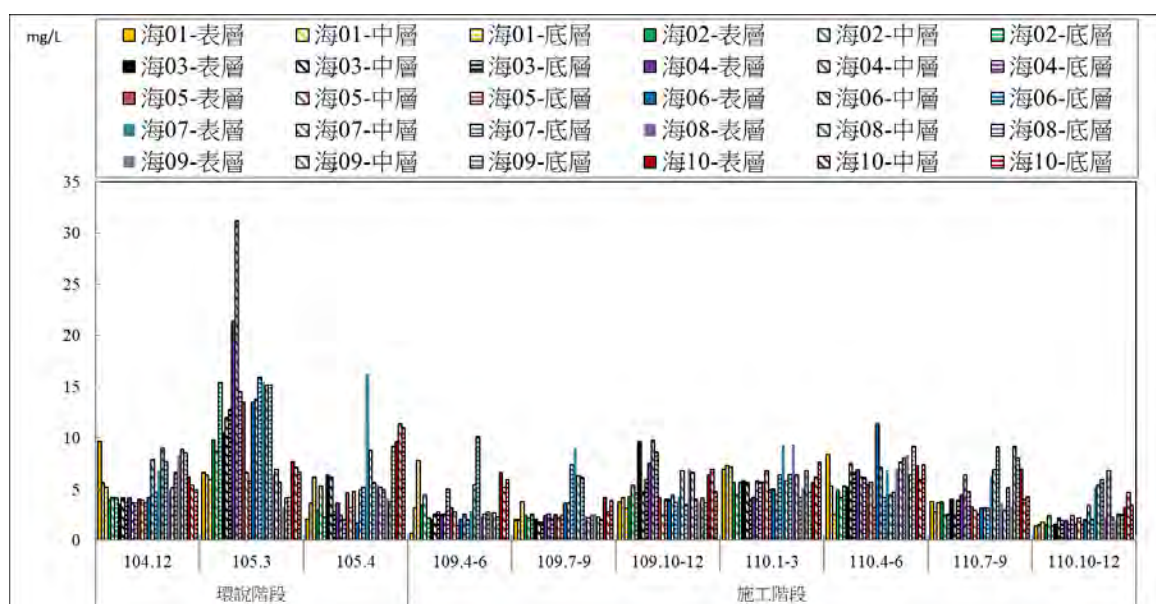
圖 3.1.7-6 歷次懸浮固體變化圖
