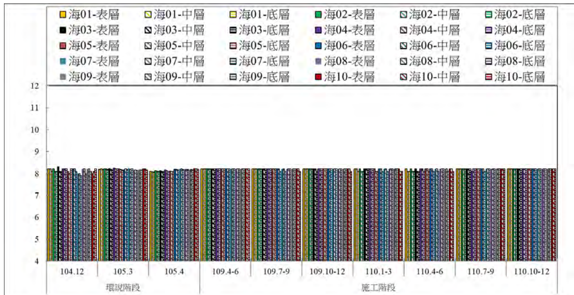
圖 3.1.7-1 歷次 pH 值變化圖
