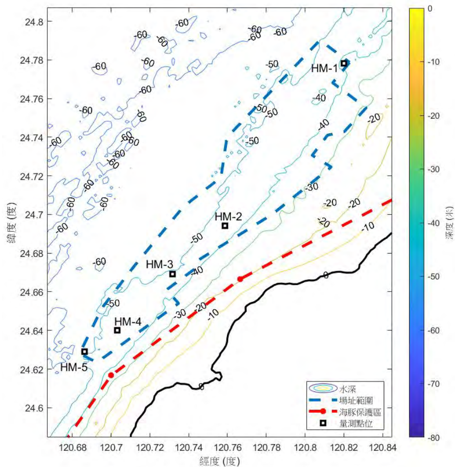
圖 1.3.3-10 水下噪音量測點位示意圖
